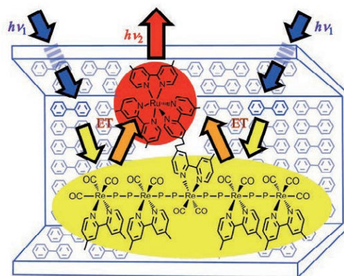
二段階光捕集系：壁に組み込んだ有機分子が吸収した光エネルギーがレニウムポリマーを経由して、最終的に全てレニウム錯体に集約される
