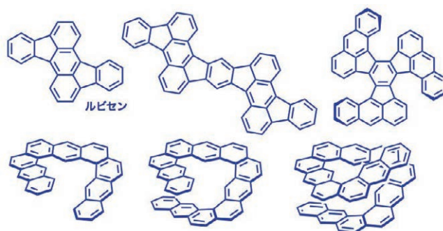
図4 \pi 共役系拡張多環芳香族化合物
