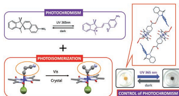
図3. 可視光・紫外光で変化するフォトクロミックコバルト錯体有機フォトクロミズム+コバルト錯体の結晶相光異性化反応（左図）、その場フォトクロミズム制御を行う新規錯体の結晶構造（右上図）とフォトクロミック色変化（右下図）
