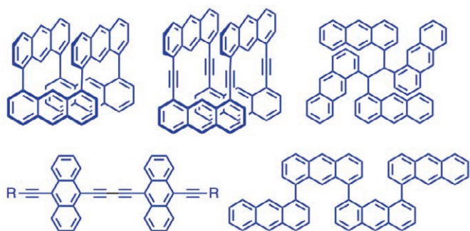
図2 研究室で合成された新しいアントラセン集積化合物
