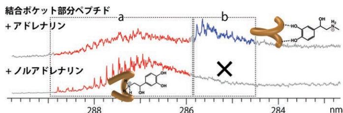
\beta 2-アドレナリンレセプターの結合ポケット部分ペプチド (SIVSF) とアドレナリンおよびノルアドレナリンとの複合体の紫外スペクトル。ノルアドレナリンは \beta 2-アドレナリンレセプターには結合しにくく、ノルアドレナリン複合体ではアドレナリン複合体で観測されるb-バンドが観測されない。このバンドは赤外分光により分子認識構造（上図）であることがわかった。
