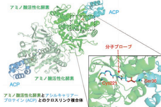
図3 クロスリンク複合体の結晶構造
