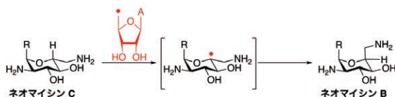
図2 ラジカル酵素による異性化機構
