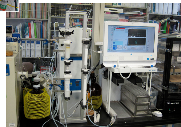
自動カラムクロマトグラフ精製装置
