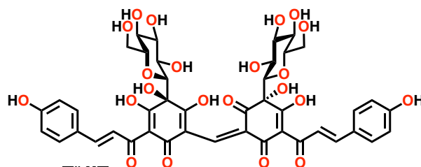
carthamin
