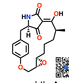
macrocidin A
