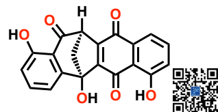
engenharquinone
