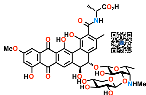
pradimicin A
