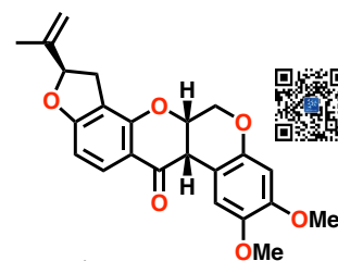
rotenone
