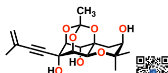
oxirapentyne D
