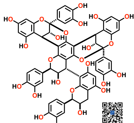
parameritannin A2
